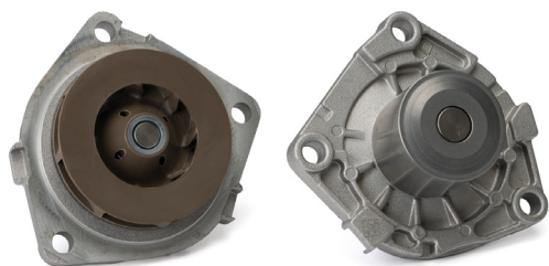
Снимка 1: 538 0310 10 - охлаждаща помпа със стандартен лагер
