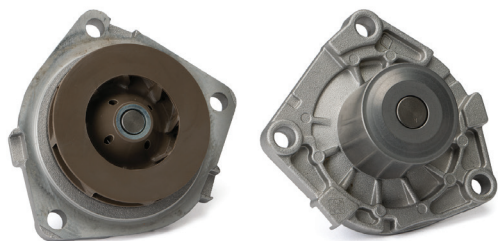
Kuva 1: 538 0310 10 - Jäähdytysnestepumppu standardilaakerilla
