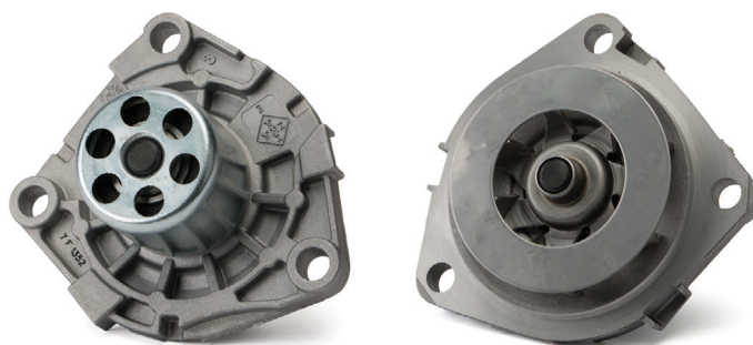
Kuva 2: 538 0714 10 - Jäähdytysnestepumppu vahvistetulla ulkolaakerilla
