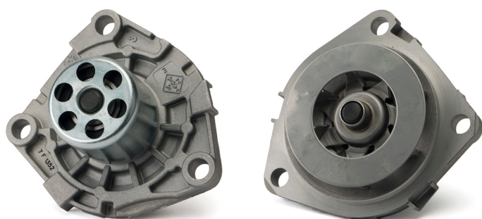
איור 2: 538 0714 10 – משאבת מים בעלת מיסב משופר, מיסב חיצוני
