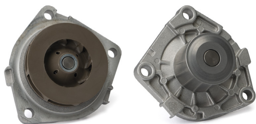
1. ábra: 538 0310 10 - vízpumpa hagyományos csapággal
