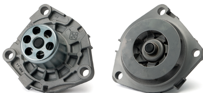
Figura 2: 538 0714 10 – pompă de apă cu rulment exterior ranforsat
