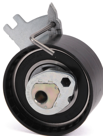
Εικόνα 2: Τροποποιημένος τεντωτήρας 531 0885 10
