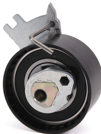
2. ábra: Módosított feszítőgörgő 531 0885 10
