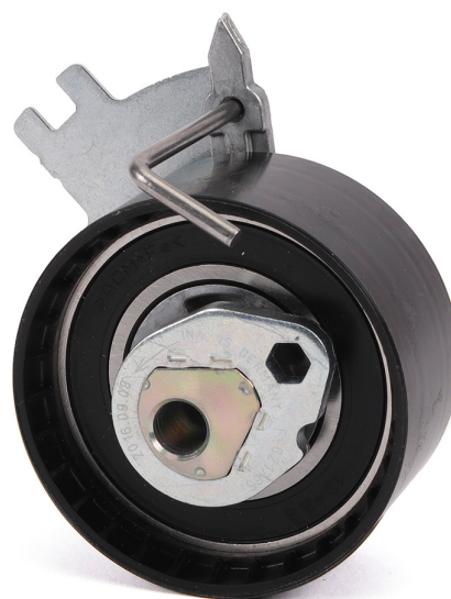
Fig. 2: Fulie întinzător modificată 531 0885 10
