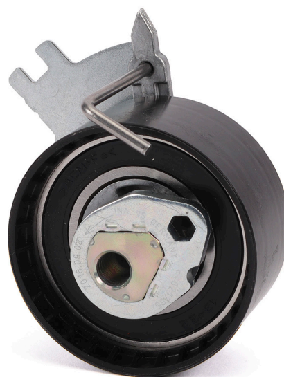
Bild 2: Modifierad spännrulle 531 0885 10
