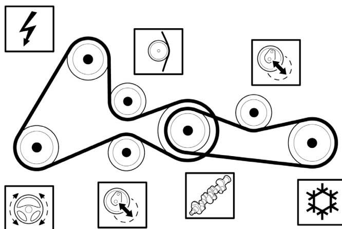
Снимка 1: Аксесоарно задвижване до номер на двигателя 0103089 с обтяжна ролка
