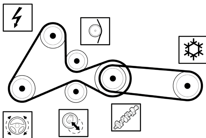
Obrázek 2: Pohon přídatných agregátů od čísla motoru 0113090 s elastickým klínovým žebrovaným řemenem
