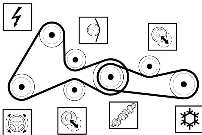
Obrázek 1: Pohon přídatných agregátů do čísla motoru 0113089 s napínací kladkou
