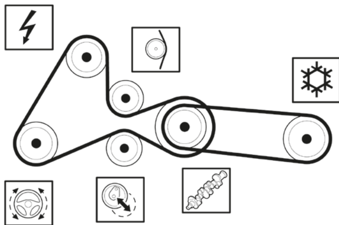
Εικόνα 2: Διάταξη εξωτερικού ιμάντα, από τον Αρ. κινητήρα 0113090 με ελαστικό ιμάντα Poly-V
