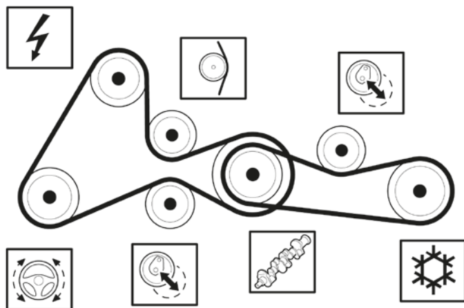
Εικόνα 1: Διάταξη εξωτερικού ιμάντα, μέχρι τον Αρ. κινητήρα 0113089, με τεντωτήρα
