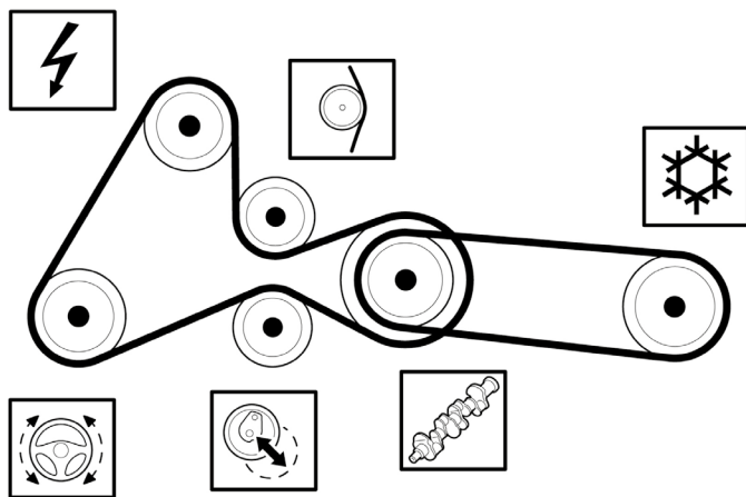
איור 2: מערכת רצועת מנוע החל ממנוע מספר: 0113090 בעלת הרצועה האלסטית.
