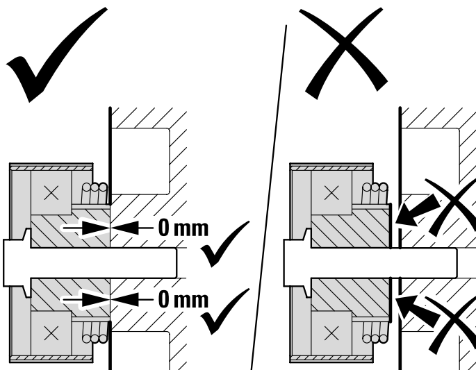
Kuva 2: Vasemmalla - kiristinpyörä koskettaa koko pinnallaan asennuspintaa moottorissa Oikealla - kiristinpyörä ei kosketa koko pinnallaan asennuspintaa moottorissa
