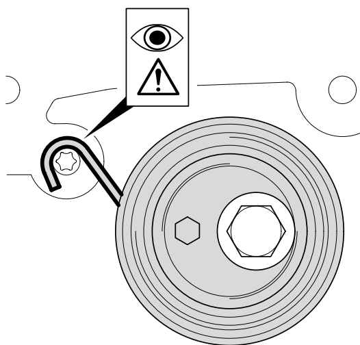
1. ábra: A rugó korrekt beszerelési helyzete a rögztőtűskén
