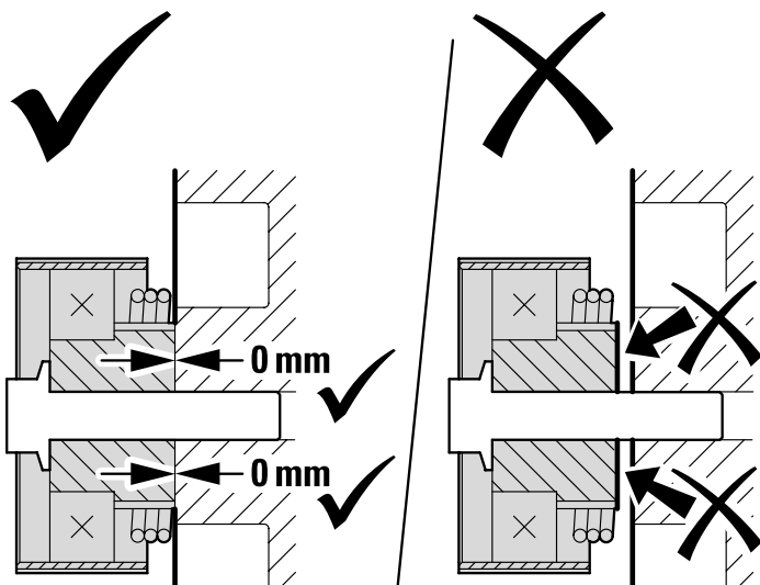
Fig. 2: Stânga – Rola întinzătorului este în contact cu întreaga suprafață de montare a sa pe motor. Dreapta – Rola întinzătorului nu este în contact cu întreaga suprafață de montare a sa pe motor.
