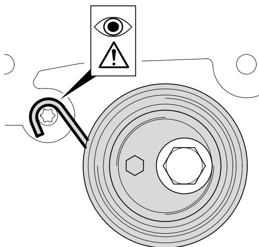
Bild 1: Korrekt monteringsläge hos fjädern på fästskruven
