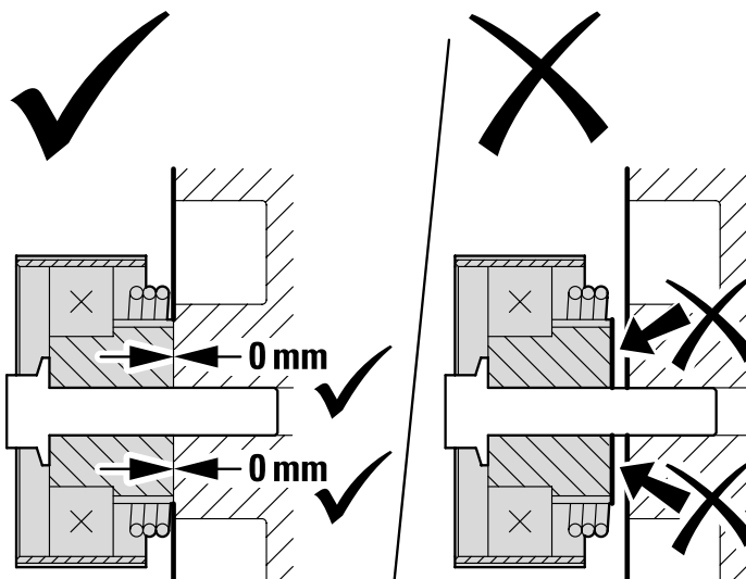
Bild 2: Vänster - spännrullen är monterad med hela ytan liggande an mot motorns fästytta Höger - spännrullen är inte monterad så att hela ytan ligger an mot motorns fästytta
