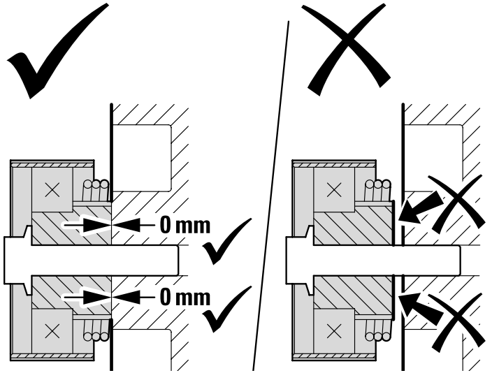
Resim 2: Sol – Gergi makarası motorun montaj yüzeyinin tamamına temas eder Sağ – Gergi makarası motorun montaj yüzeyinin tamamına temas etmez
