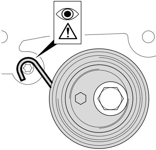
Resim 1: Yayın ankraj civatasına doğru şekilde takılması
