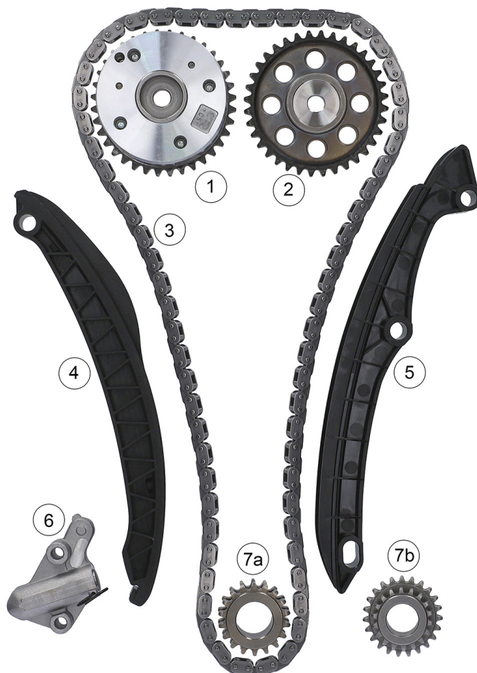
Снимка 1: 559 0154 30/559 0154 31 – Компоненти за комплект ангренажна верига
