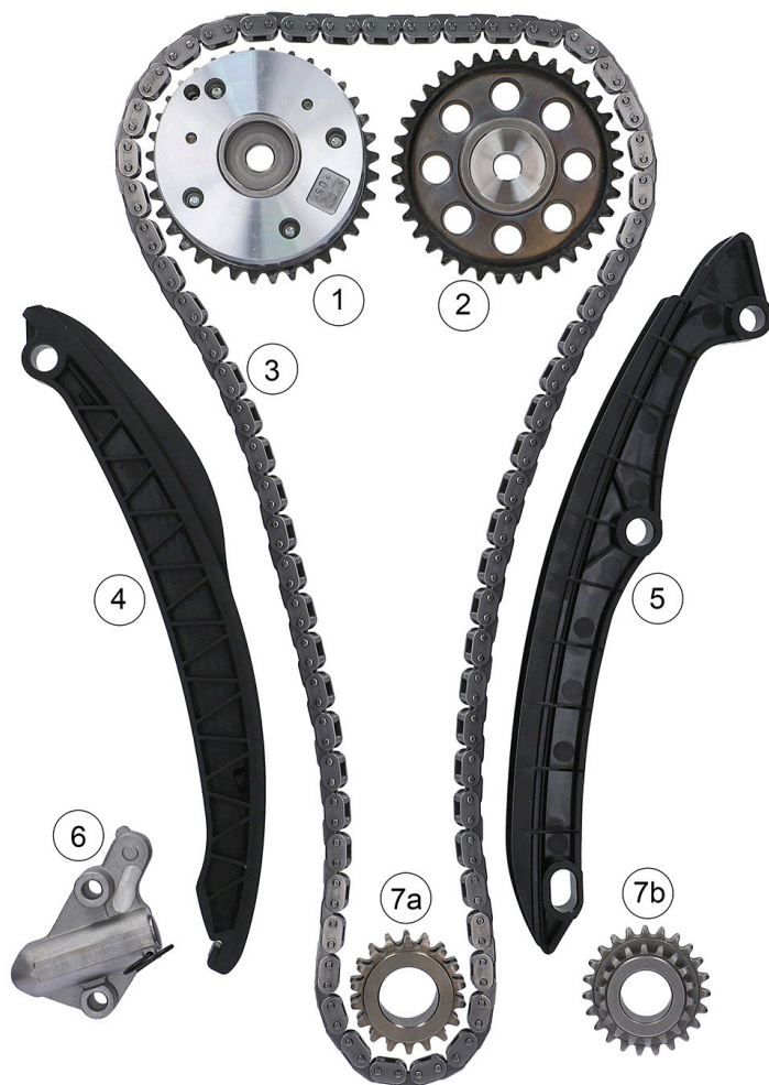
Obrázek 1: 559 0154 30/559 0154 31 – konstrukční díly sada rozvodového řetězu
