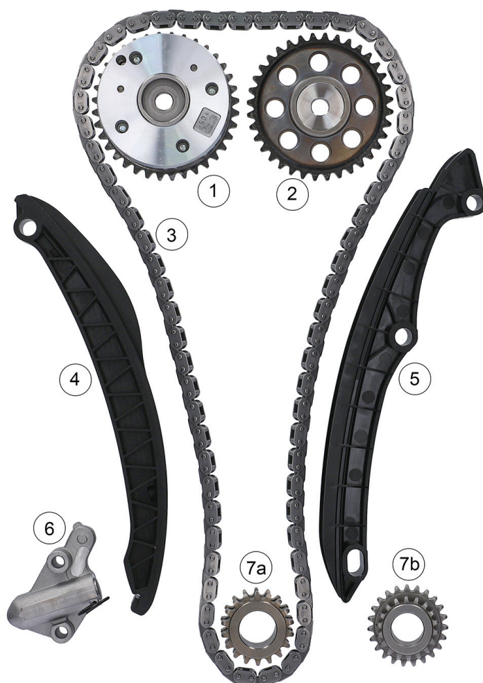
Figuur 1: 559 0154 30/559 0154 31 – onderdelen distributieketting-KIT
