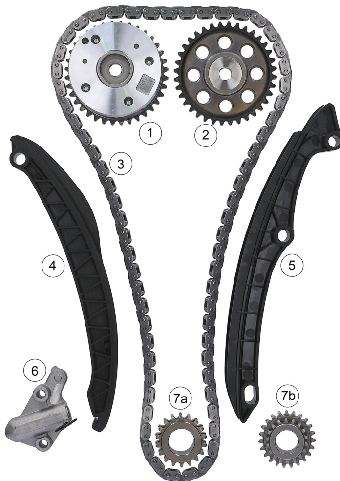
Fig. 1: 559 0154 30/559 0154 31 – Componente KIT lanț de distribuție
