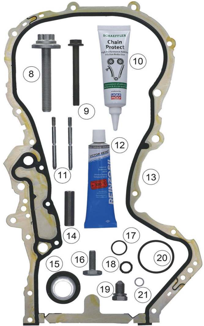
Resim 2: 559 0154 30/559 0154 31 - Zamanlama zinciri kiti ek parçaları
