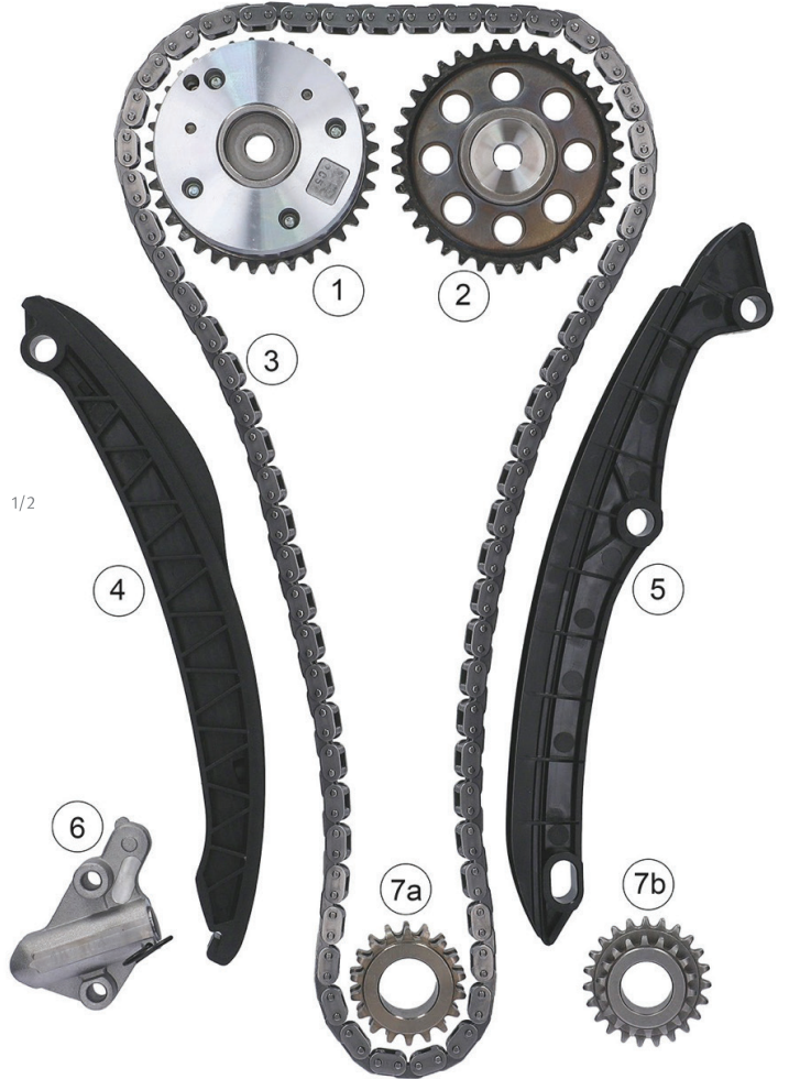
Resim 1: 559 0154 30/559 0154 31 – Zamanlama zinciri kiti bileşenleri
