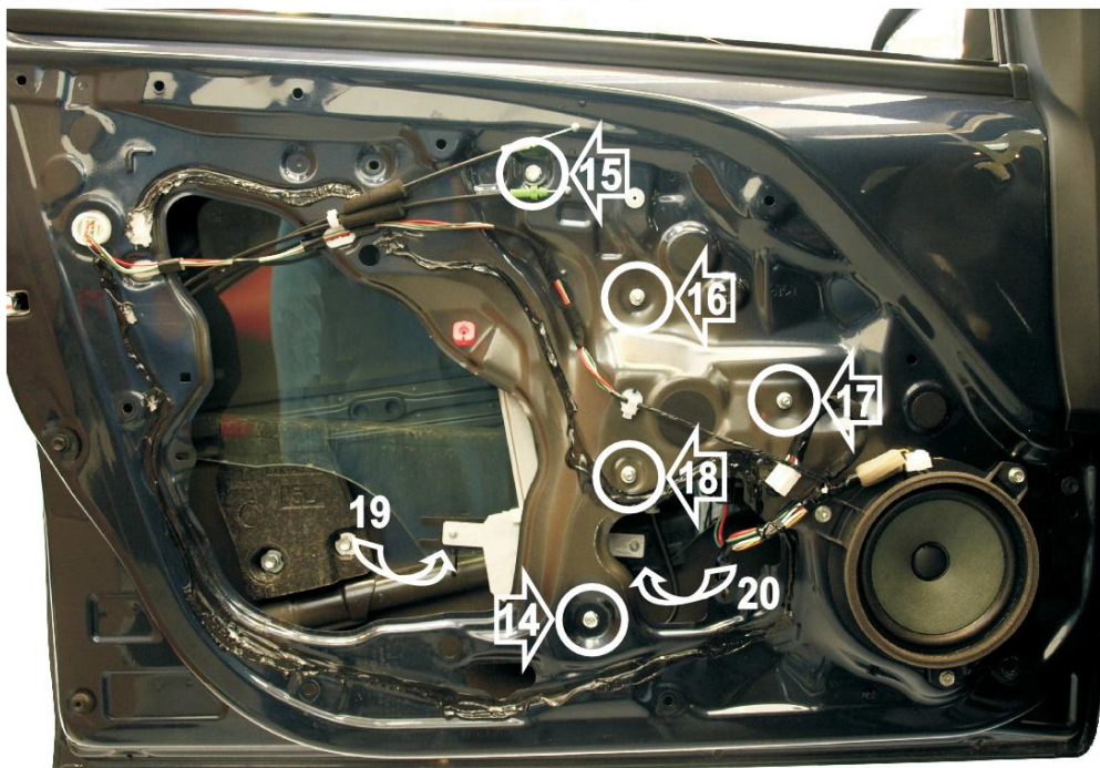
Porta lato sinistra- Left hand side door
