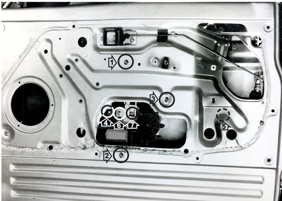
Porta lato destro - Right hand side door
