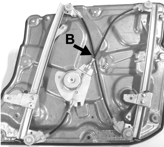
Porta lato sinistro - Left hand side door
