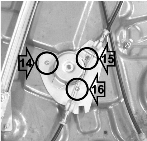
Porta lato sinistro - Left hand side door
