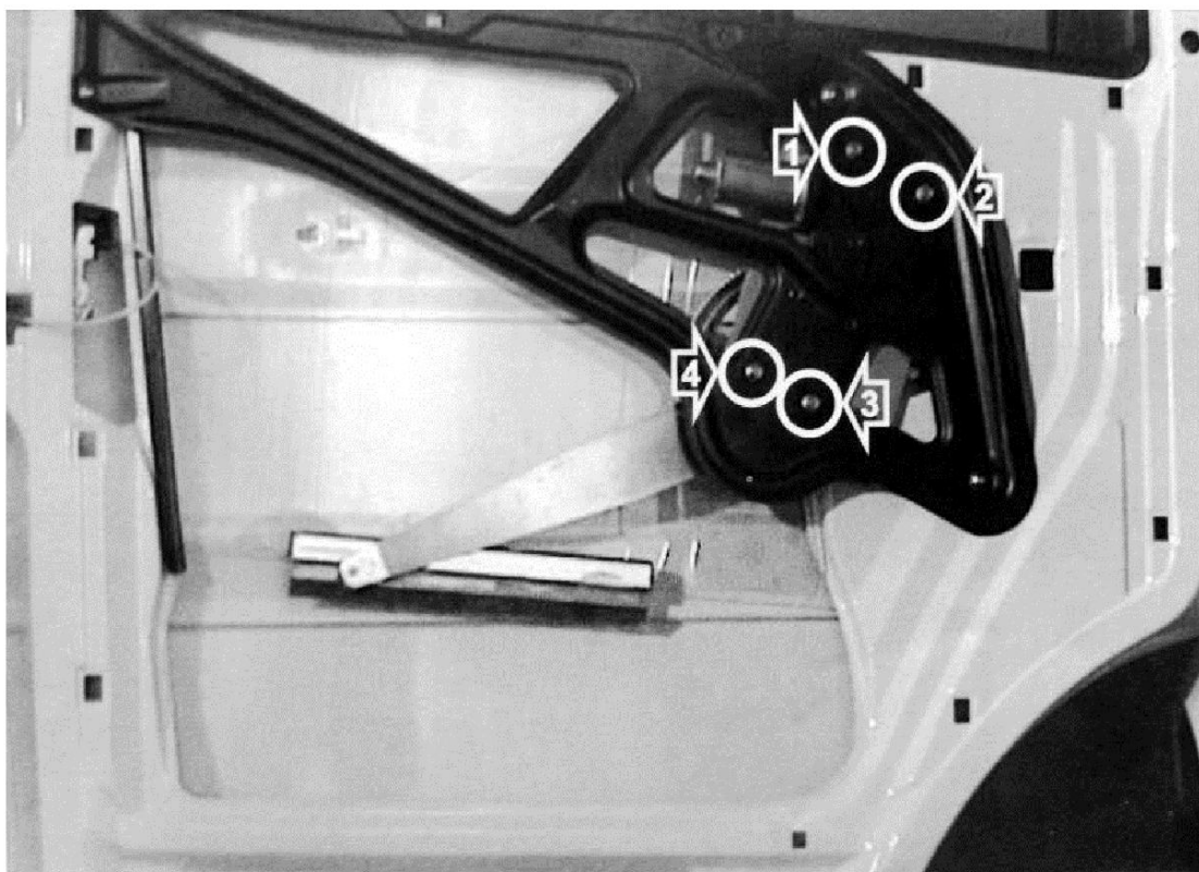
Porta lato sinistra - Left hand side door
