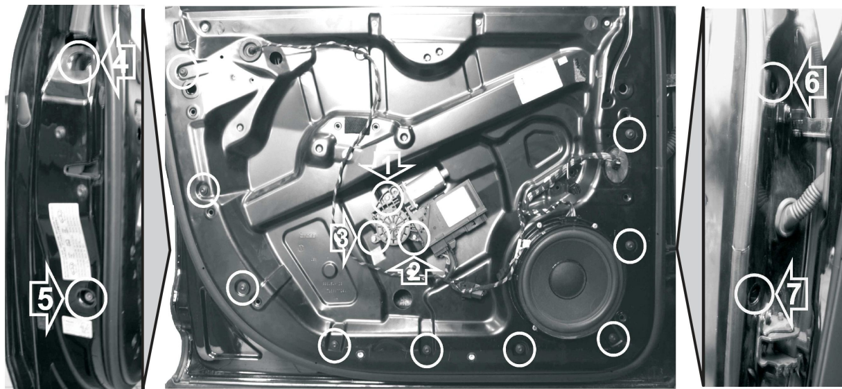
Porta lato sinistra- Left hand side door
