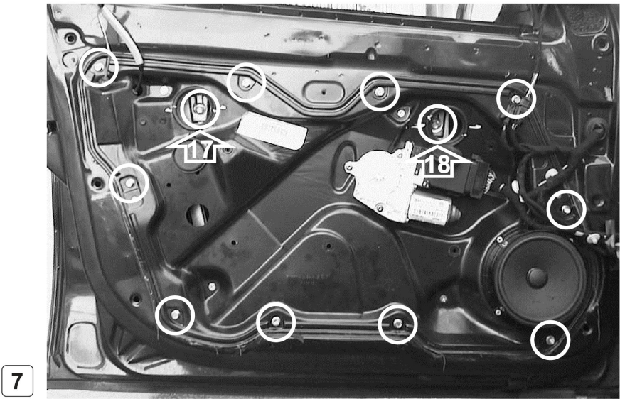
Porta lato sinistra - Left hand side door
