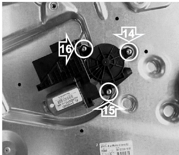
Porta lato sinistro - Left hand side door
