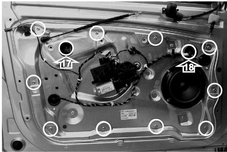
Porta lato sinistro - Left hand side door
