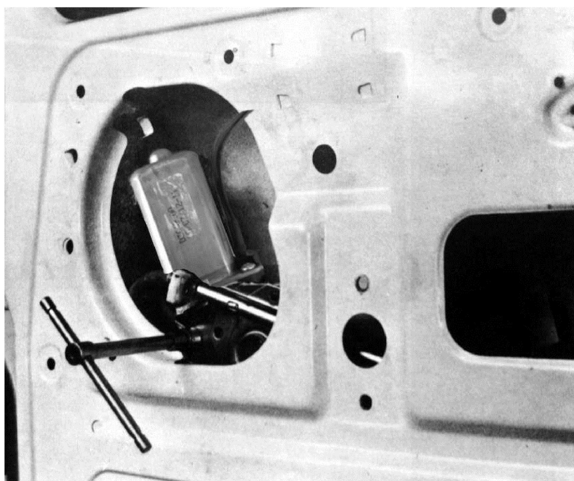
Porta lato destro - Right hand side door
