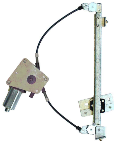
POWER WINDOW RIGHT ALZACRISTALLI ELETTRICO DX
