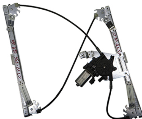
POWER WINDOW RIGHT ALZACRISTALLI ELTTRICO DX
