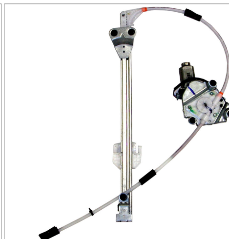
ORIGINAL POWER WINDOW LEFT ALZACRISTALLI ELETTRICO ORIGINALE SX
