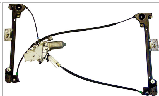
ORIGINAL POWER WINDOW ALZACRISTALLI ELETTRICO ORIGINALE
