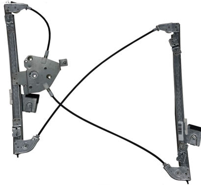
POWER WINDOW LEFT ALZACRISTALLI ELETTRICO SX
