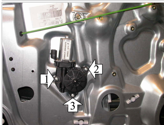
MOTOR LEFT MOTORE SX
