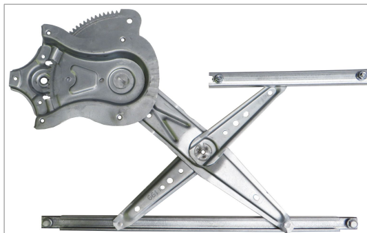
POWER WINDOW RIGHT ALZACRISTALLI ELETTRICO DX
