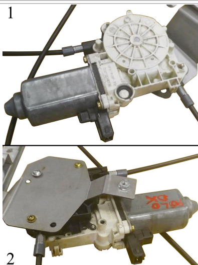
POWER WINDOW LEFT ALZACRISTALLI ELETTRICO SX
