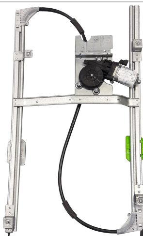
POWER WINDOW RIGHT ALZACRISTALLI ELETTRICO DX
