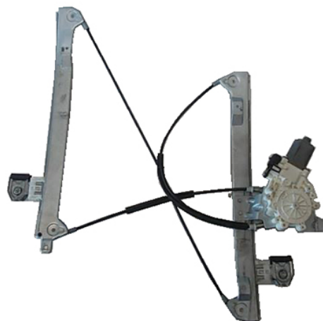
ORIGINAL POWER WINDOW LEFT ALZACRISATLLI ELETTRICO ORIGINALE SX
