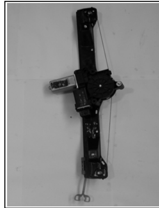
Alzacristallo originale – oem window regulator – lève-vitre original – Fensterheber von oem – elevalunas original – levandator de vidro original – orijinal cam acacagi – Γρύλος γνήσιος
