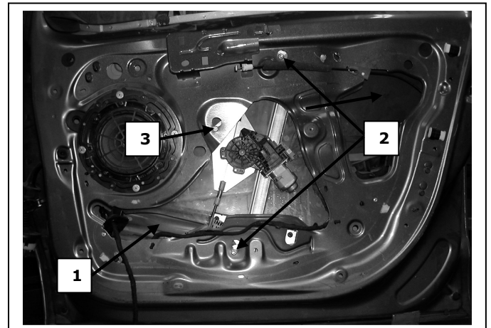
Porta lato destro, Portière avant droite, Right front door, Puerta lado derecho, Vorne rechte Tür, Porta frente dirieta, Sag on kapi, νόρτα εμπρόςθια δεξιά
