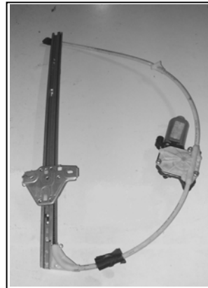
Alzacristallo originale – oem window regulator – lève-vitre original – Fensterheber von oem – elevalunas original – levantador de vidrio original orijinal cam acacagi - Γρύλος γνήσιος
