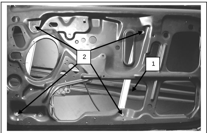
Porta lato destro, Portière avant droite, Right front door, Puerta lado derecho, Vorne rechte Tür, Porta frente dirieta, Sağ on kapi, πόρτα εμπρόςθια δεξιά
