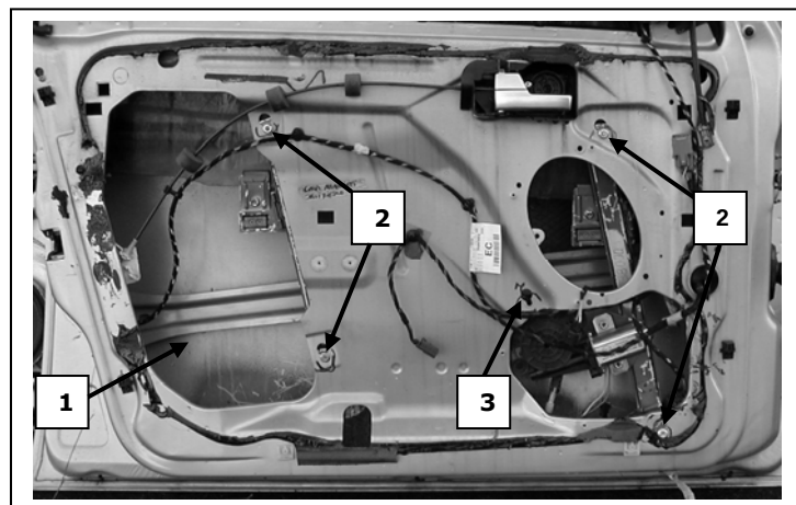
Porta lato sinistro, Portière avant gauche, Left front door, Puerta lado izquierdo, Vorne links Tür, Porta frente esquerda, Sol on kapi, πόρτα εμπρόςθια αριστερή
