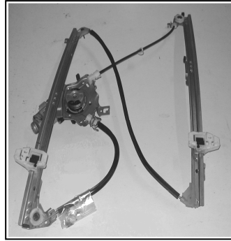
Alzacristallo originale – oem window regulator – lève-vitre original – Fensterheber von oem – elevaunas original – levandator de vidro original – bizim cam acacagi - Γρύλος γνήσιος
