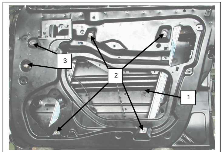
Porta lato destro, Portière avant droite, Right front door, Puerta lado derecho, Vorne rechte Tür, Porta frente dirieta, Sag on kapi, πόρτα εμπρόςθια δεξιά
