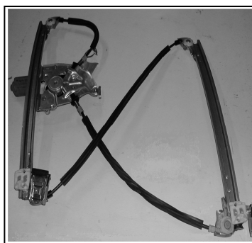
Alzacristallo originale – oem window regulator – lève-vitre original – Fensterheber von oem – elevalunas original – levantador de vidro original orijinal cam acacagi - Γρύλος γνήσιος
