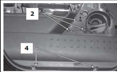
Alzacristallo originale - oem window regulator - lève-vitre original - Fensterheber von oem - elevaunas original - levandador de vidro original - orijinal cam acacagi - Γρύλος γνήσιος
